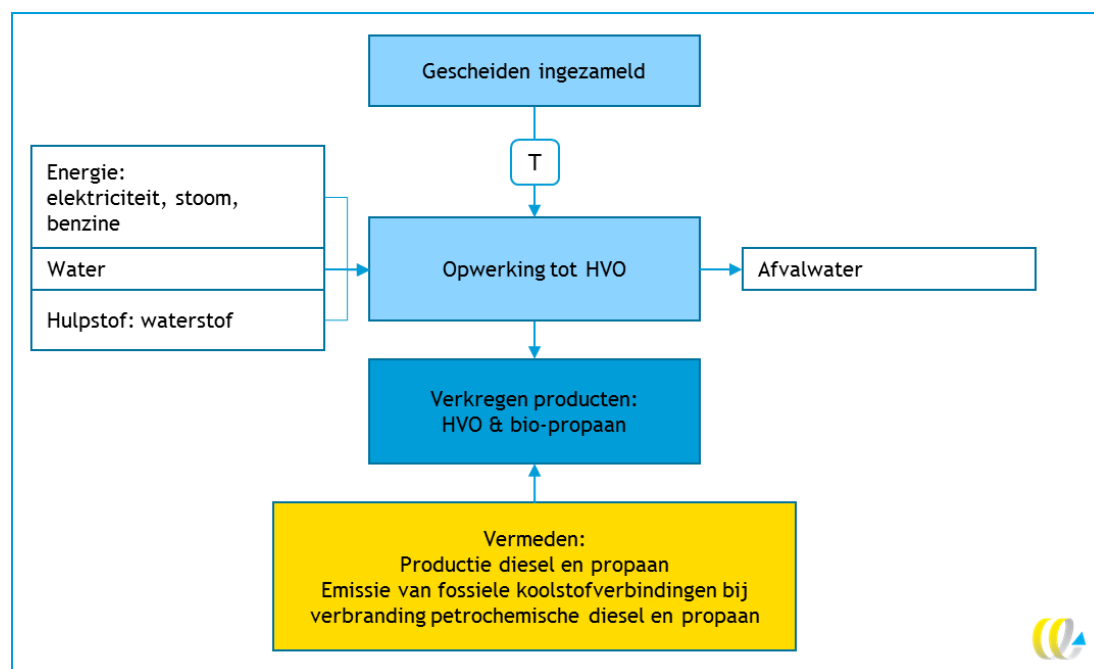
Figuur 27 - Processtappen HVO-productie van frituurolie en vet
