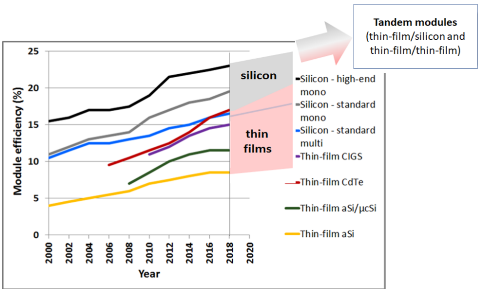
Figuur 5 – Stijgende efficiëntie van verschillende type zonnecellen sinds 2000. Bron: Wim Sinke, TNO en UvA
