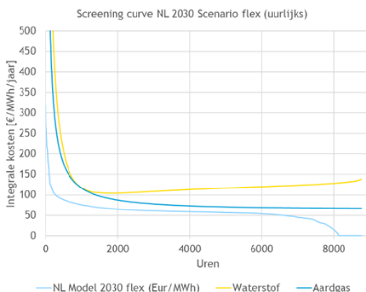
Figuur 11: Prijsduurkromme voor de waterstofketen in het flex-scenario bij een variabele waterstofprijs op basis van de elektriciteitsprijs.
