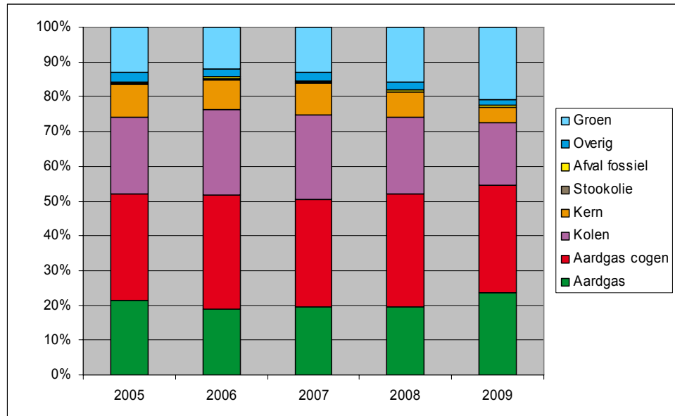
Figuur 4 Leveringsmix in 2005 t/m 2009
