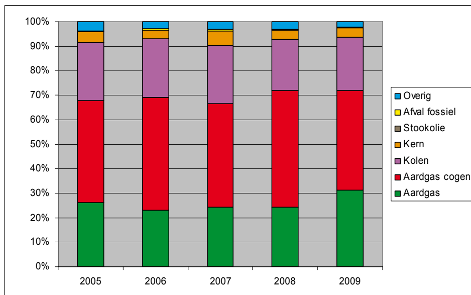
Figuur 2 Productiemix in 2005 t/m 2009
