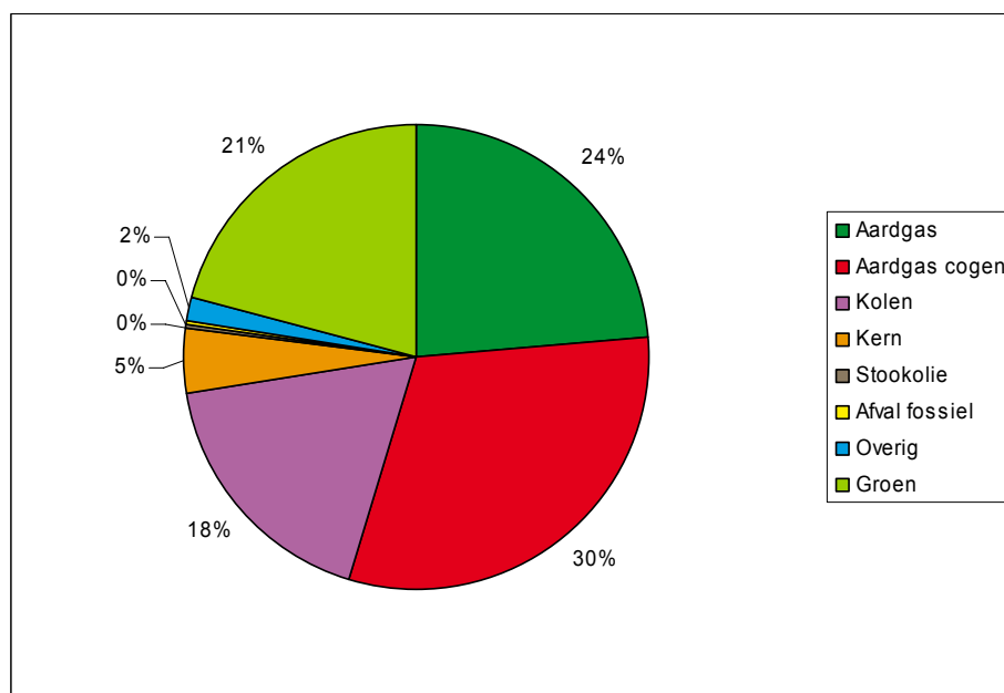
Figuur 3 Herkomst van geleverde elektriciteit in Nederland in 2009
