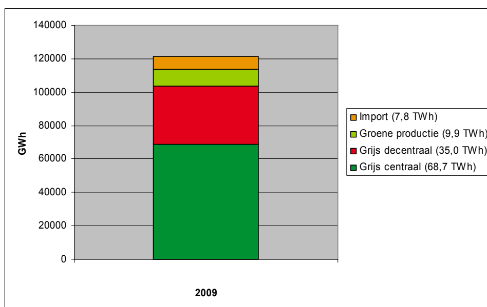
Figuur 1 Volumestromen elektriciteit Nederland 2009
