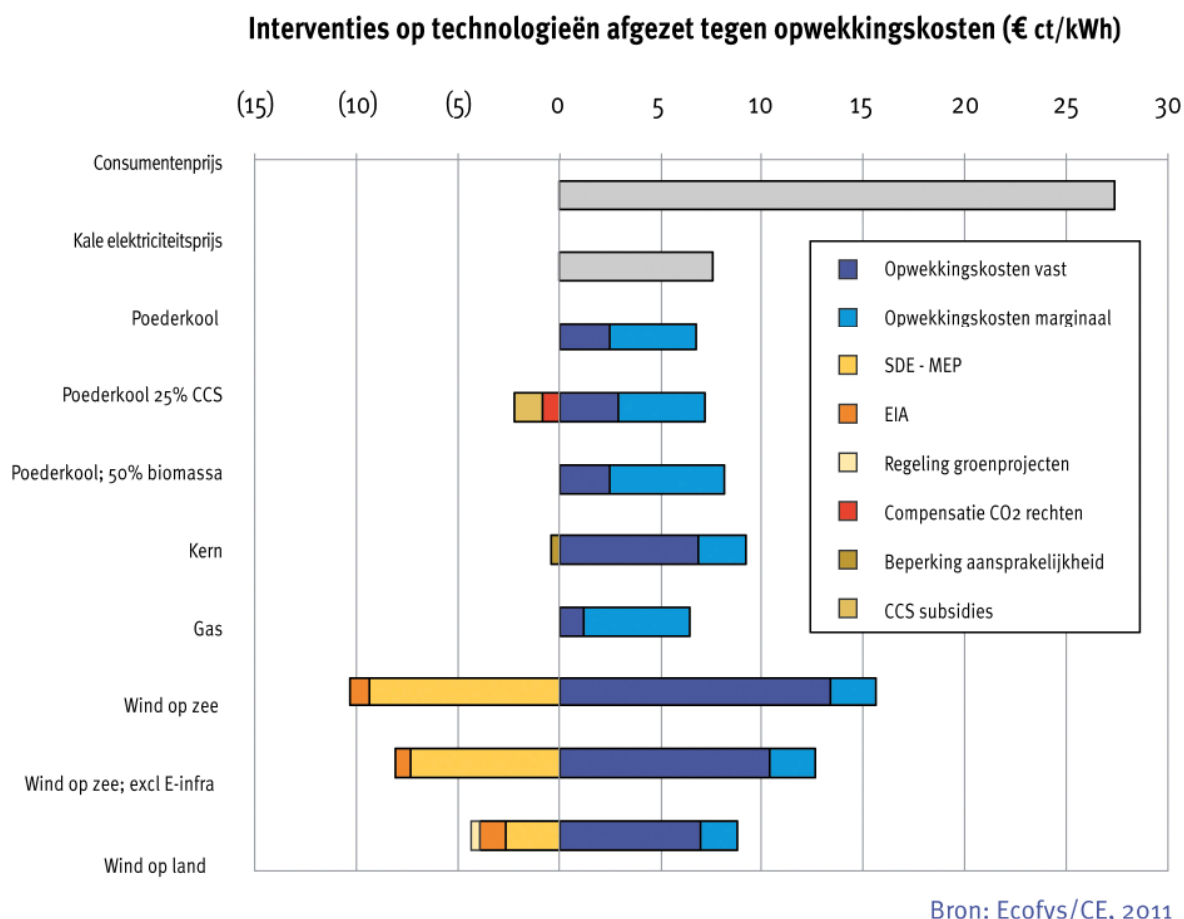
Figuur 4 - 2 Interventies op technologieën (oranje/rood) afgezet tegen de opwekkingskosten (blauw), in 2010
