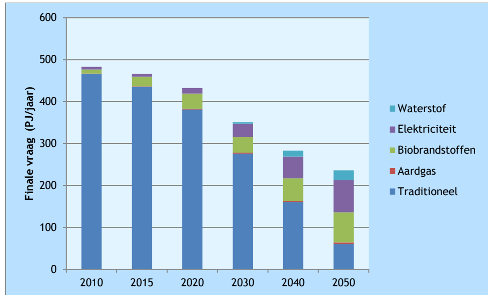
Figuur 4 Finale vraag transport in Nederland (PJ/jaar)
