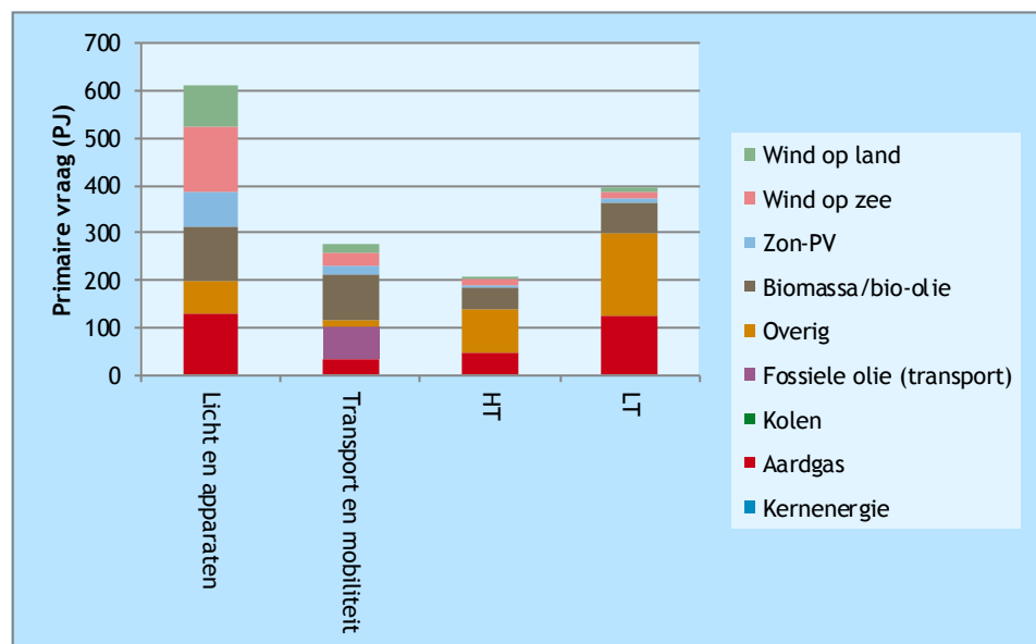
Figuur 16 Primaire vraag per functie en bron 2050 Energy (R)evolution Scenario (PJ/jaar)
