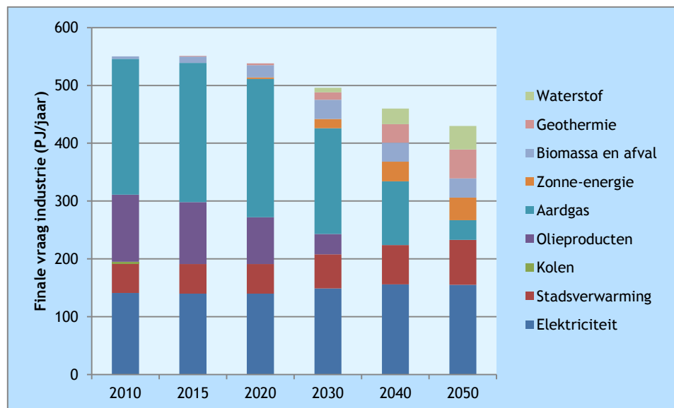
Figuur 5 Finale energievraag industrie in Nederland (PJ/jaar)
