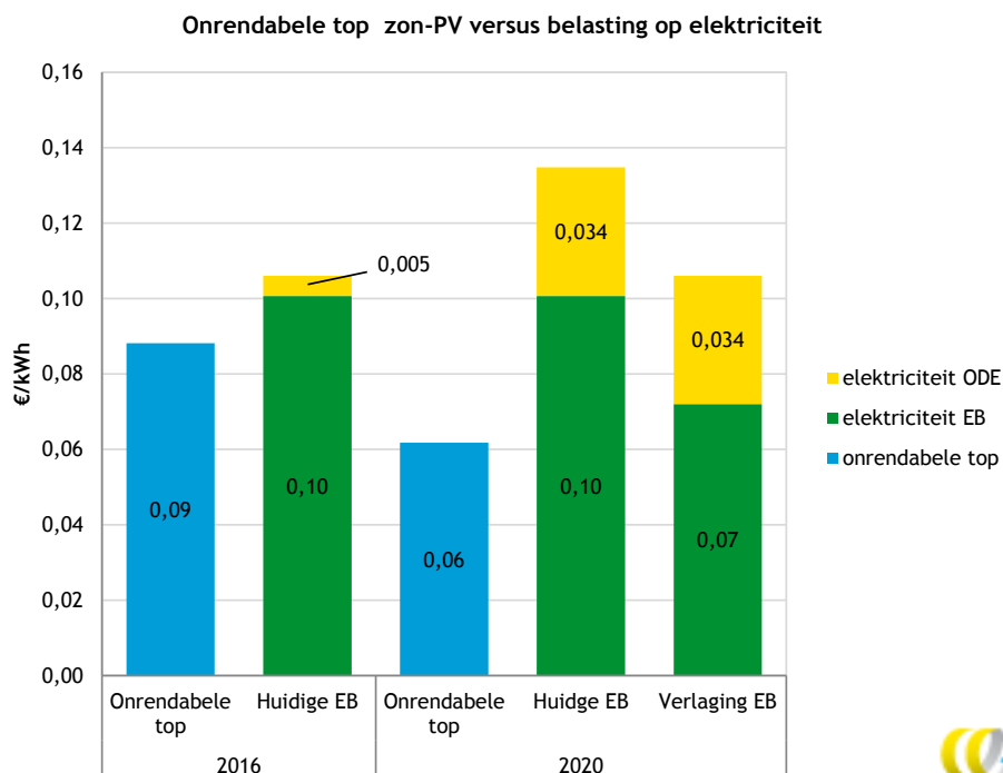
Figuur 4 Prijscomponenten zon-PV (exclusief BTW)
