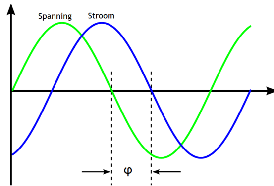
Figuur 5 Illustratie faseverschuiving
