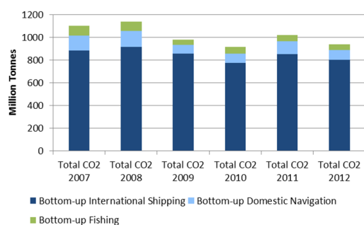
a. CO 2
