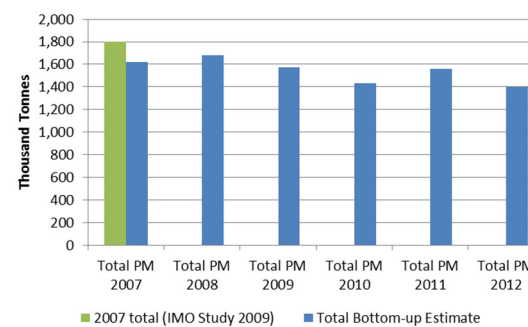
f. PM
