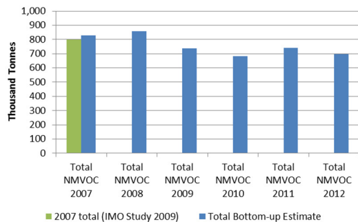
h. NMVOC
