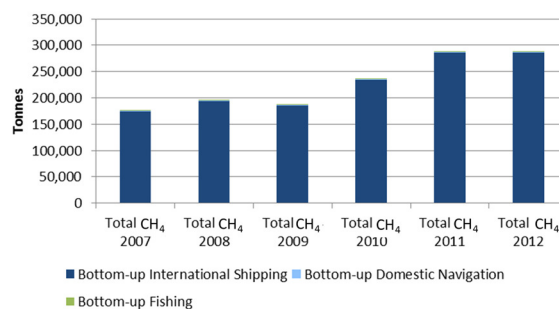
b. CH 4
