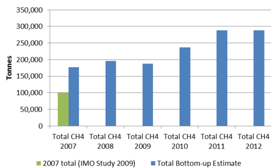
b. CH 4
