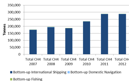
b. CH 4
