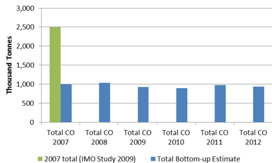
g. CO
