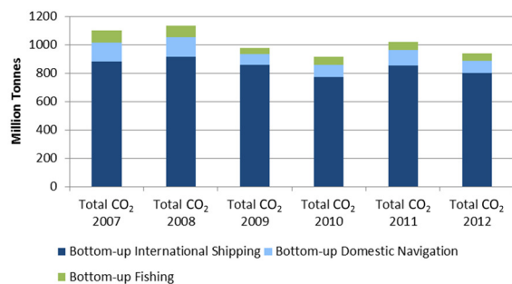
a. CO 2
