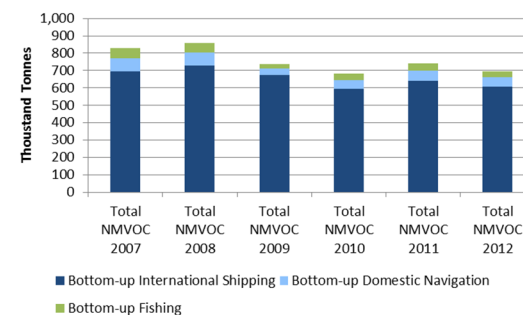
h. NMVOC
