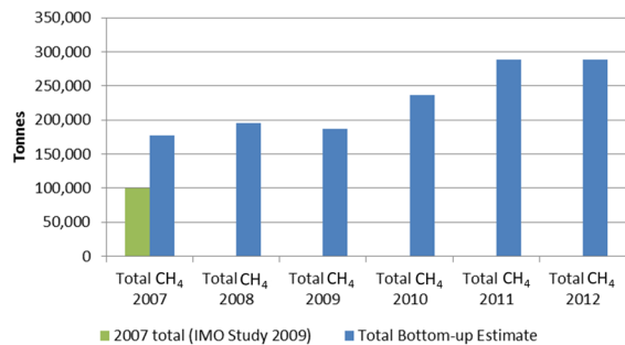
b. CH 4
