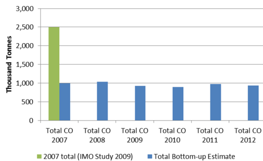
g. CO
