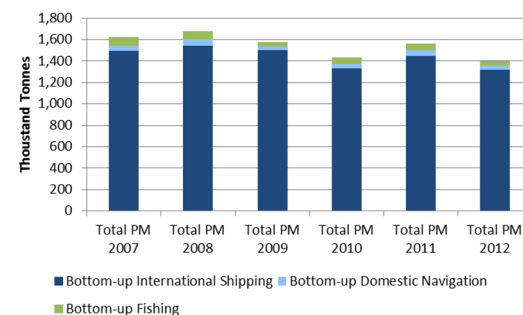
f. PM
