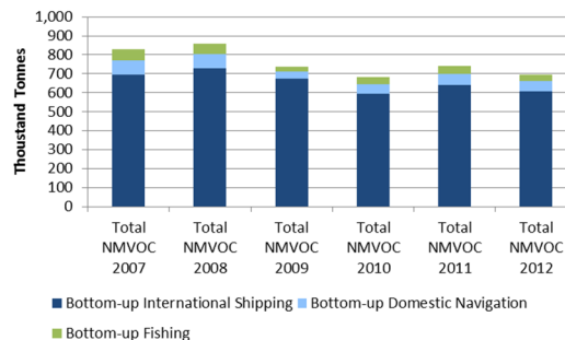
h. NMVOC
