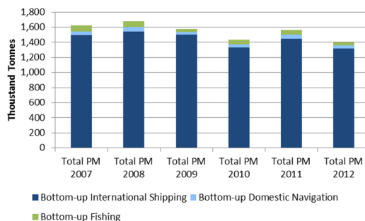
f. PM
