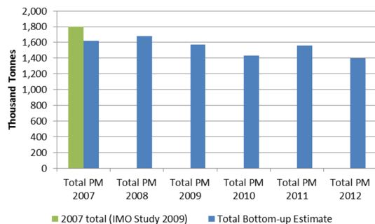
f. PM
