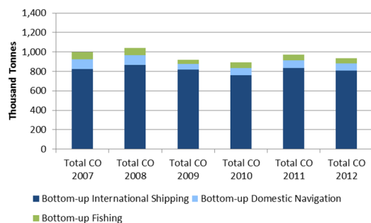
g. CO
