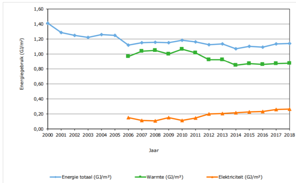
Figuur 22 - Historisch elektriciteits- en warmtegebruik in de glastuinbouw
