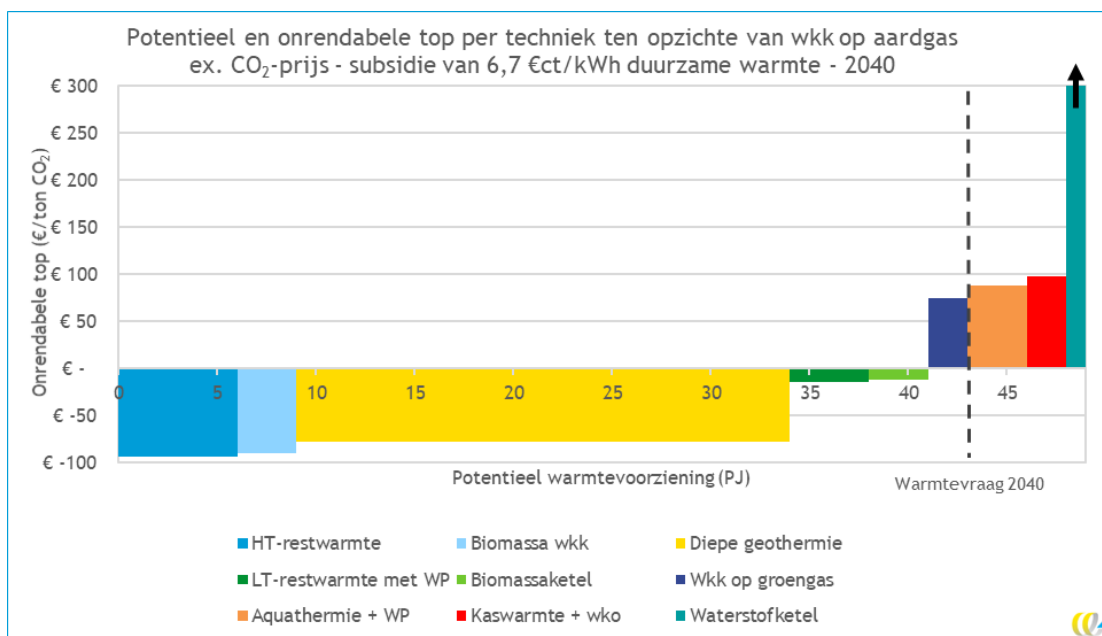
Figuur 16 - Effect van een generieke subsidie van 6,7 €ct/kWh duurzame warmte op de merit order
