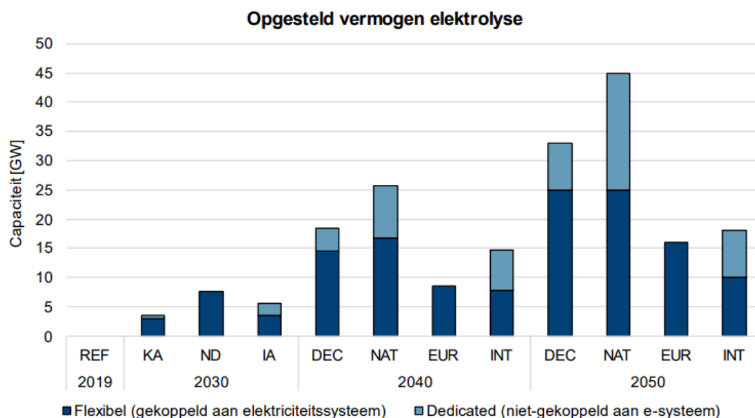
Figuur 6 - Opgesteld vermogen elektrolyse volgens scenario's in IJ3050
