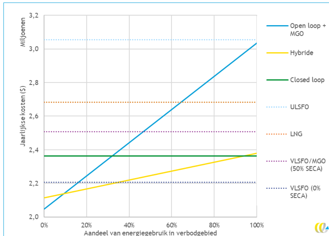
Figuur 21 - Jaarlijkse kosten van EGCS en brandstoffen voor totale brandstofverbruik bij verboden op lozen van waswater voor nieuwbouw general cargo-schip van 10.000-19.999 dwt (energieverbruik 155 TJ/jaar)
