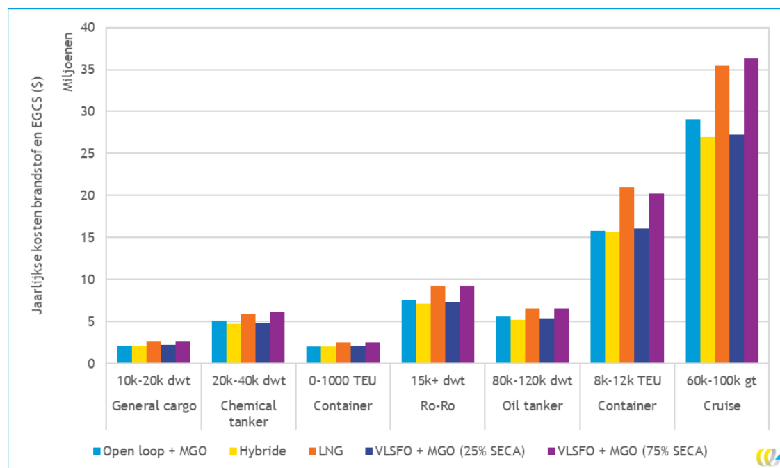
Figuur 19 - Jaarlijkse kosten voor volledig brandstofverbruik voor verschillende scheepstypen bij wereldwijd verbod lozen waswater in territoriale wateren binnen 3 nm
