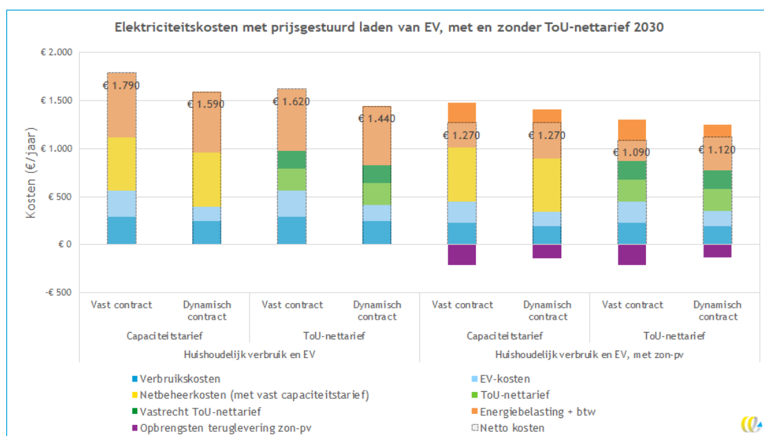
Figuur 12 - Elektricietskosten met een EV die prijsgestuurd laadt, voor vaste netbeheerkosten en een ToU-nettarief in 2030
