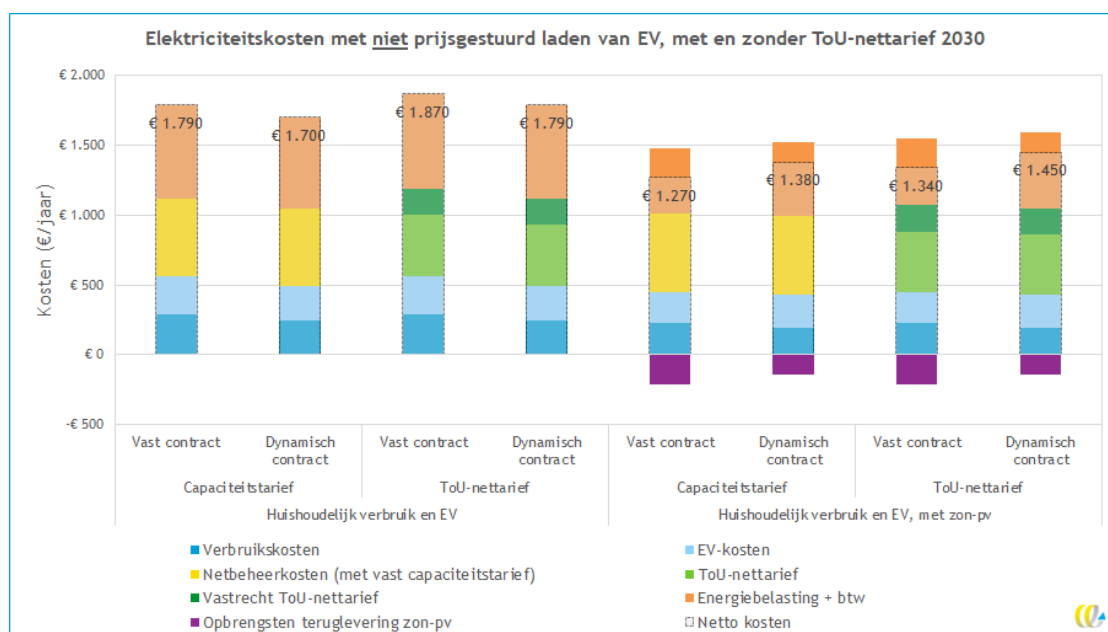
Figuur 11 - Elektricietskosten met een EV die niet prijsgestuurd laadt, voor vaste netbeheerkosten en een ToU-nettarief in 2030
