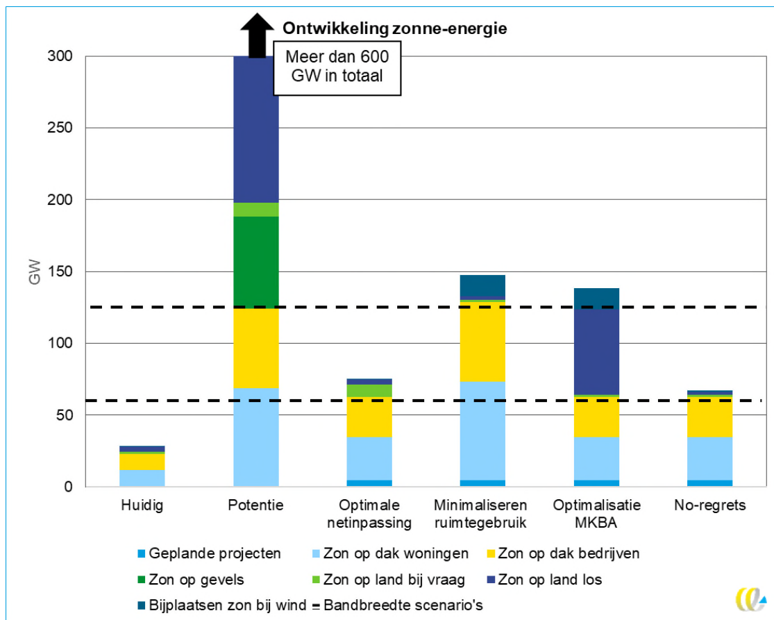
Figuur 1 – Mogelijke ontwikkelingen van zonne-energie voor de verschillende ontwikkelpaden. De stippelijnen geven de onder- en bovengrens van onderzochte scenario's voor zonne-energie in 2040.
