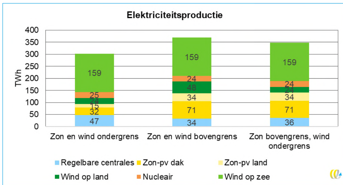
Figuur 3 – Productie elektriciteit
