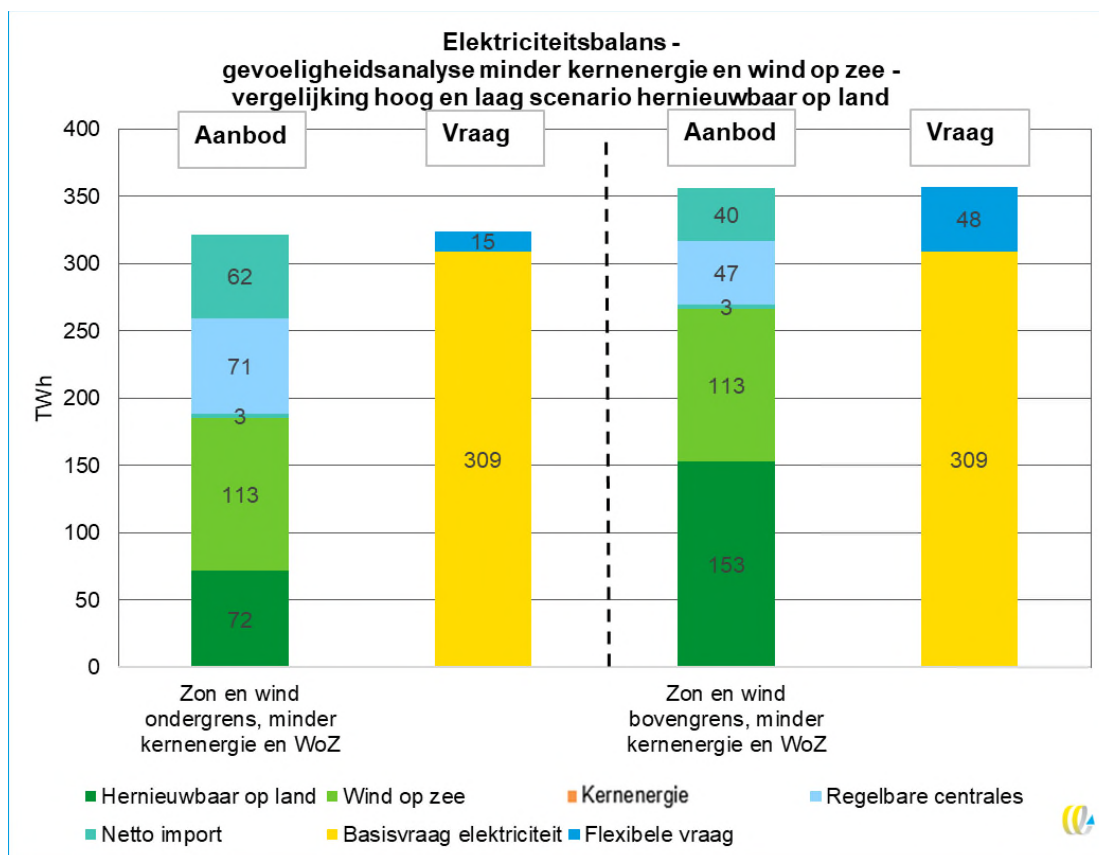
Figuur 9 – Elektricietsbalans, vergelijking ondergrensscenario en bovengrensscenario hernieuwbare opwek op land – gevoeligheidsanalyse minder kernenergie en windenergie op zee.
